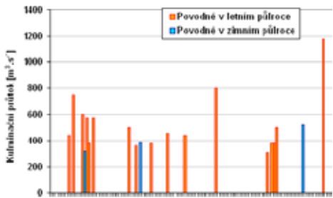
Výskyt povodní s průtokem větším než Q5 na Otavě od roku 1880. Na grafu je patrné nepravidelné rozložení povodní v čase.
