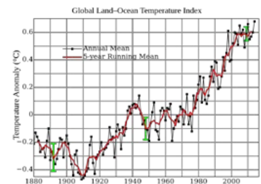
Nárůst průměrné světové teploty od roku 1880 do 2014 vtažen k průměru 1951-1981. Černá čára roční průměr, červená čára pětiletý průměr. Zdroj NASA GISS.
