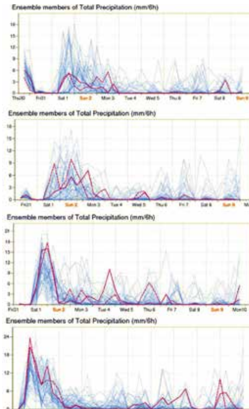
Ansámblová předpověď srážek v mm za 6 hodin z ECMWF pro Prahu na 10 dní, shora dolů: z 30. 5. 14:00, z 31. 5. 02:00, z 31. 5. 14:00 a z 1. 6. 02:00 2013. Modré čáry – jednotlivé ansámblové předpovědi, přerušovaná červ. čára – předpověď hlavního modelu, plná červená čára – předpověď kontrolního modelu.
