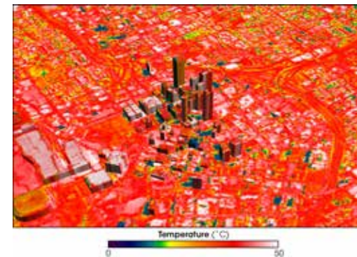
Města v letních měsících vytvářejí tzv. teplotní ostrovy, kdy je jejich teplota výrazně vyšší než okolní krajiny. To má vliv nejenom na kvalitu života v nich, ale i na odpar vody. Snímek Atlanty termokamerou v létě.
