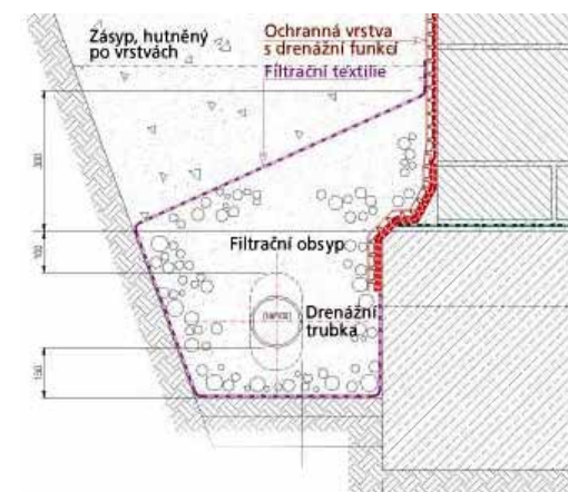
Drenáže (odvodnění) základů proved'te ve spádu.
